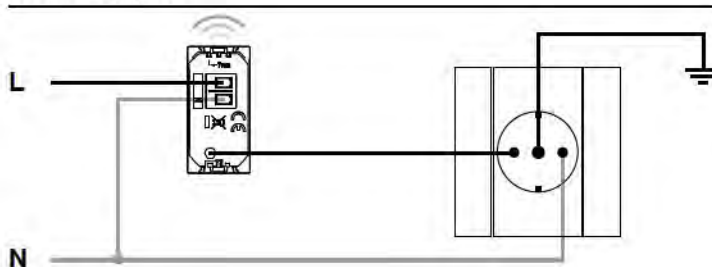
Schéma zapojenia
